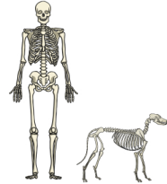
skeletons
