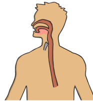
oesophagus
